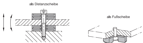
Montagebeispiele
